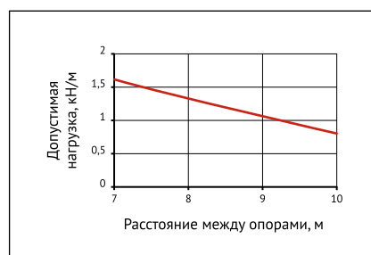
Диаграмма нагрузок на кабельный лоток
