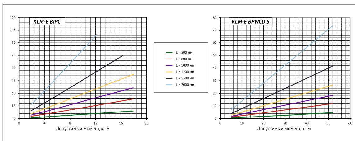
График нагрузок. KLM-E BIPC и KLM-E BPWCD 5
